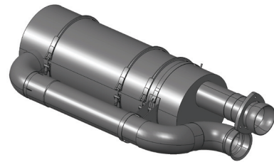
Systeme zur Nachrüstung des Volvo FL6 mit D6B Motor ABE 17181 zum Euro 3 mit 184kW
